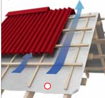
Неутепленная крыша
