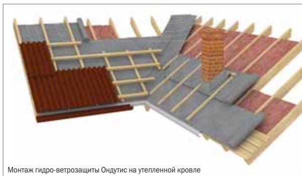
Монтаж гидро-ветрозащиты Ondutis на утепленной кровле
